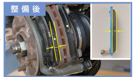
ブレーキ・パッドが新品の状態
