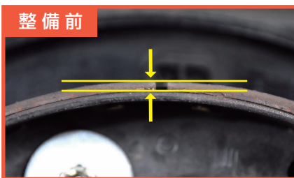
ブレーキ・シュー(ライニング)が減っている状態
